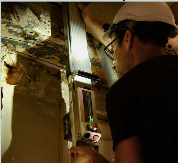
Títol: "Anàlisi resistogràfica de la fusta"
